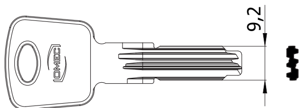
SCALA 1:1
